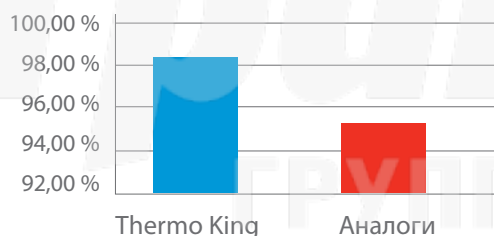
Эффективность удаления эмульгированной воды
